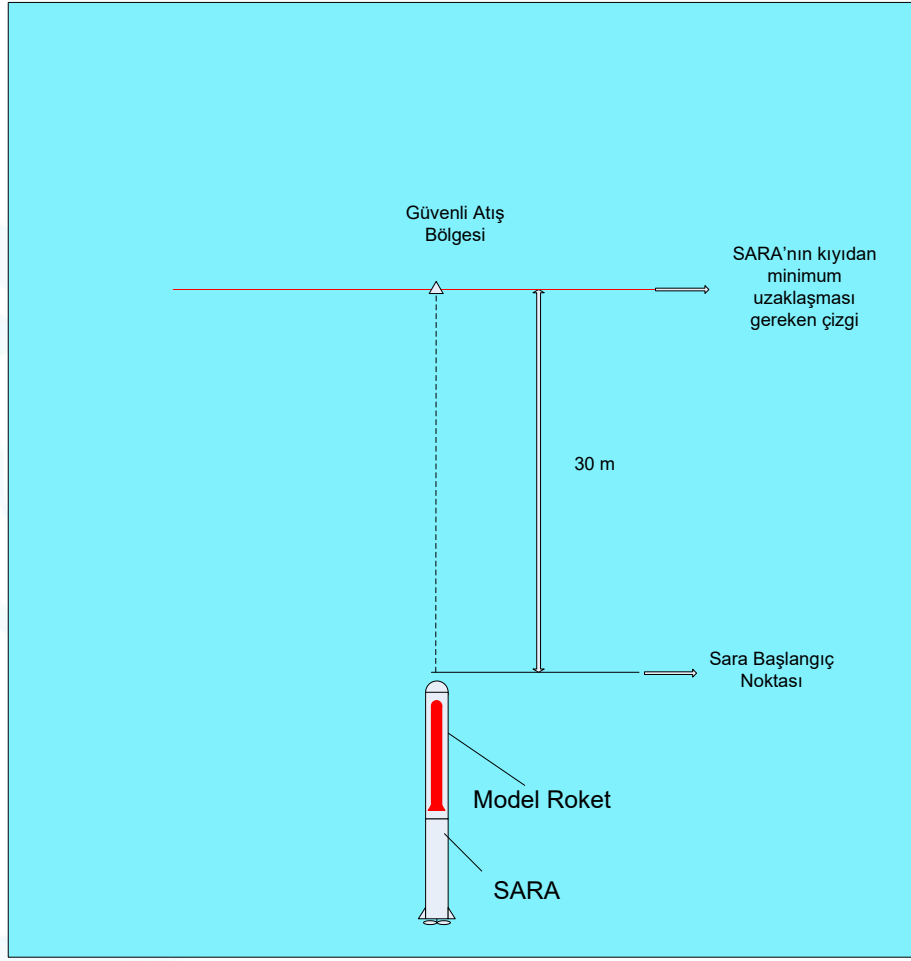
Figure 3 Aşama 2 - Temsili Üstten Gösterim
